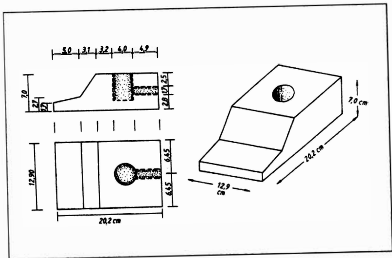
Рис. 1. Эскиз предмета из Аюда с размерами.
