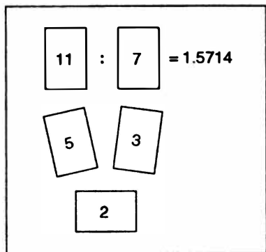
Рис. 1. Простые числа. Аппроксимация половины числа симметрии 3.14159.
