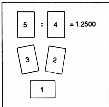
Рис. 2. Натуральные числа. Аппроксимация половины числа фикуса 2.5029.
