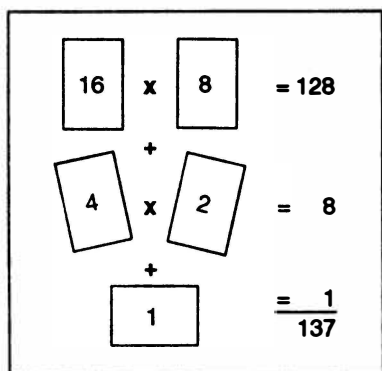
Рис. 3. Двоичные числа. Аппроксимация констант микроструктуры 137.036.
