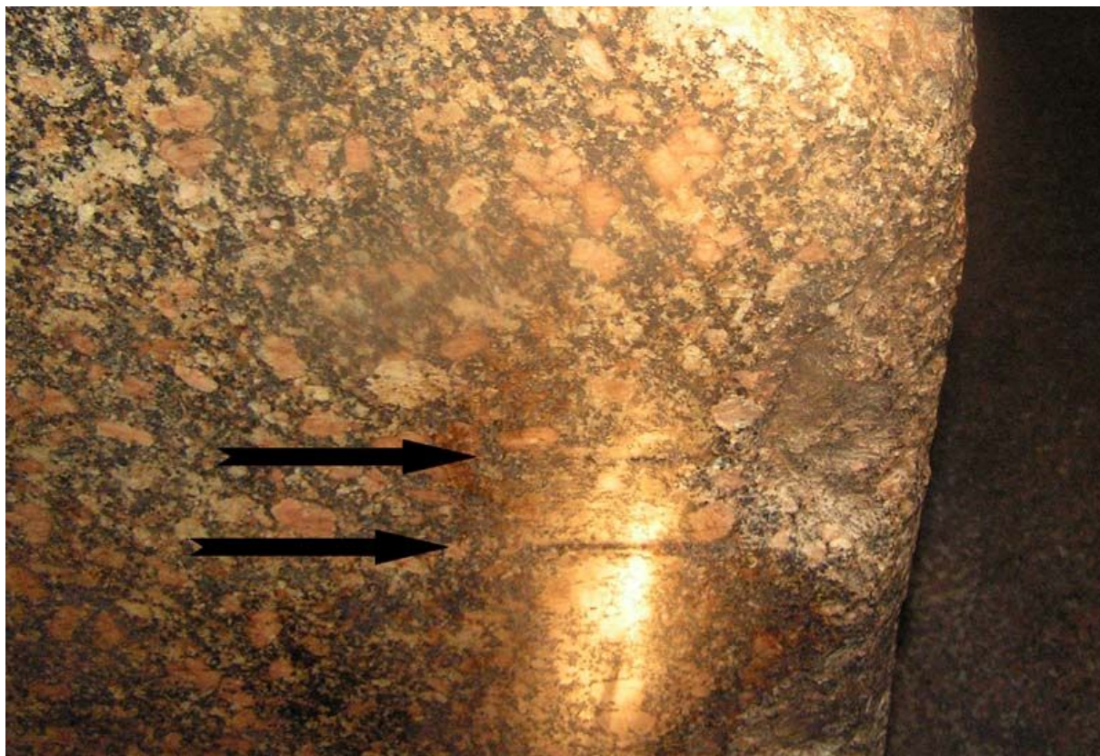
Рис. 56. Следы от пилы на «саркофаге» в Великой пирамиде
