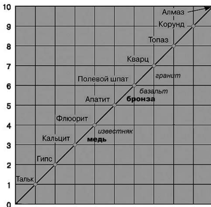
Рис. 47. Шкала Мооса
