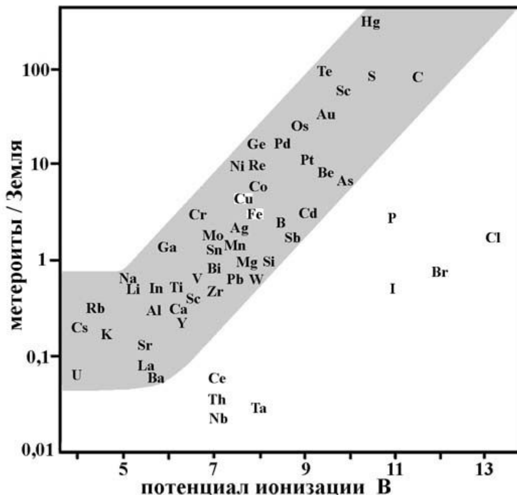
Рис. 182. Распространенность элементов в метеоритах
