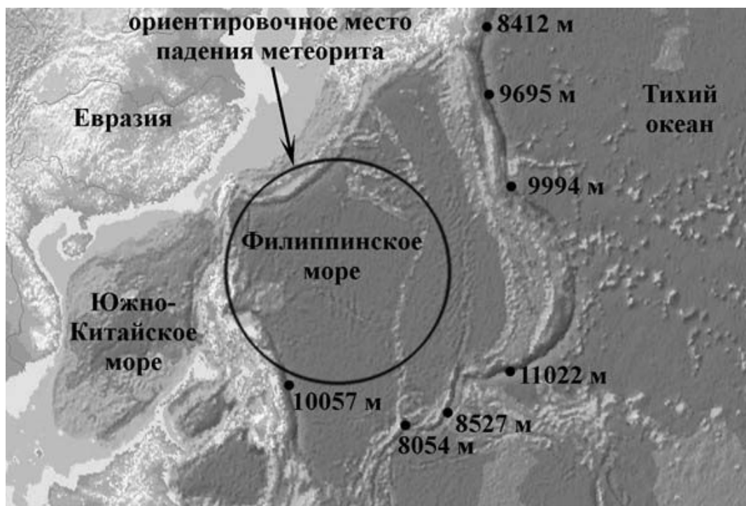
Рис. 8. Физическая карта Филиппинского моря.
