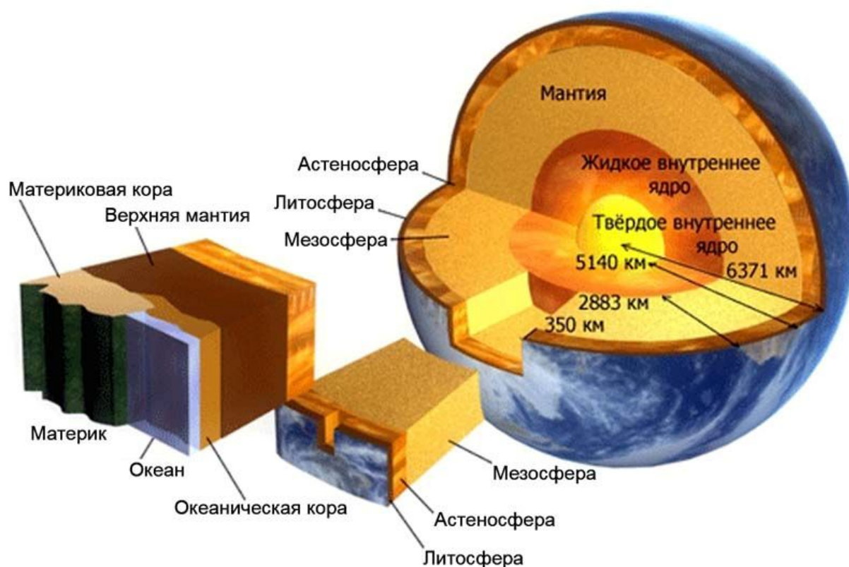
Рис. 4. Строение Земли
