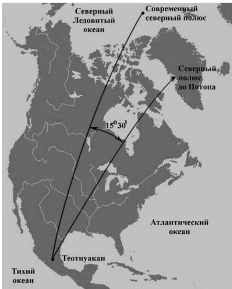
Рис. 38. Определение допотопного положения Северного полюса
