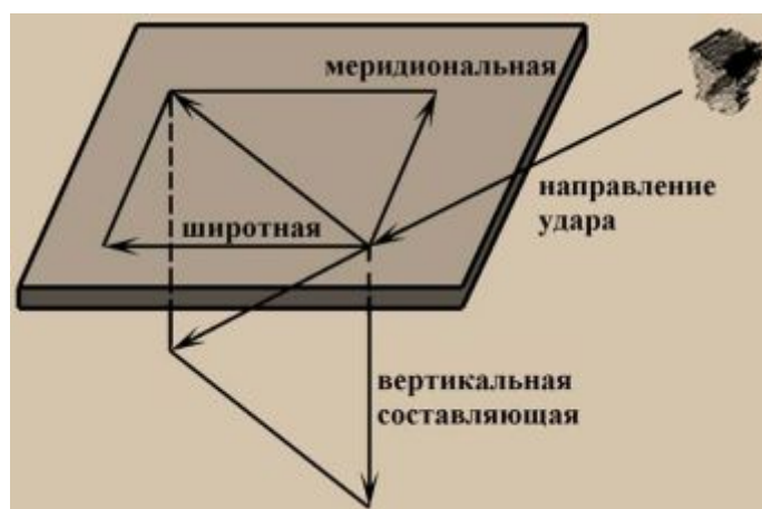
Рис. 5. Составляющие силового воздействия при падении метеорита
