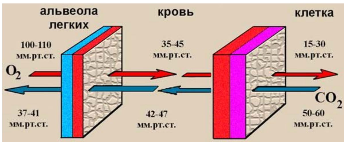
Рис. 179. Транспорт газов.
