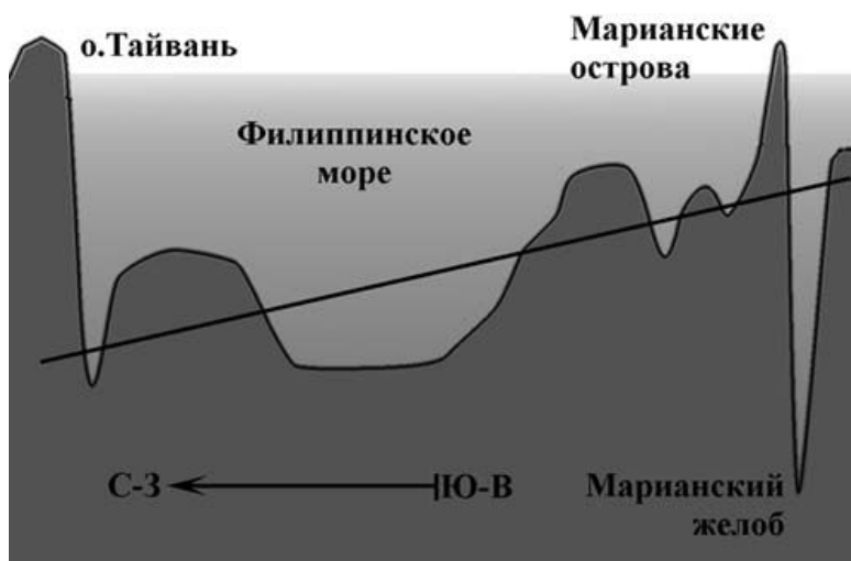
Рис. 9. Профиль дна Филиппинского моря
