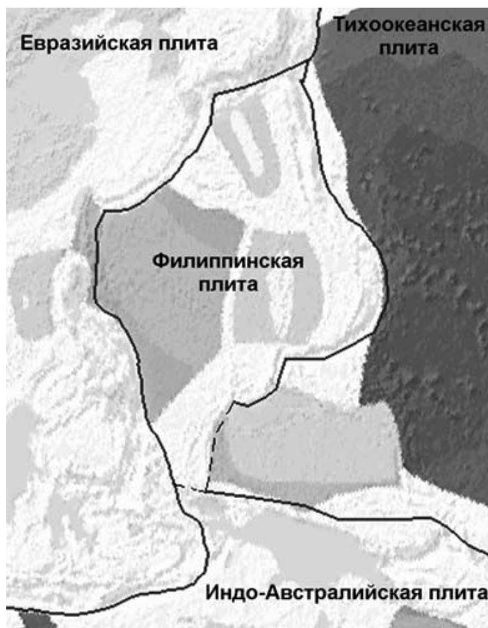
Рис. 7. Тектоническая карта района Филиппинского моря.
